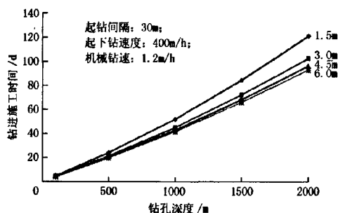
图1 回次长度对钻进施工时间的影响
