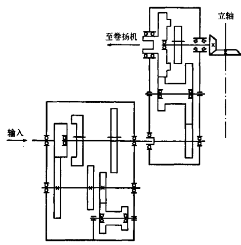
图 4 改进后的传动系统图
