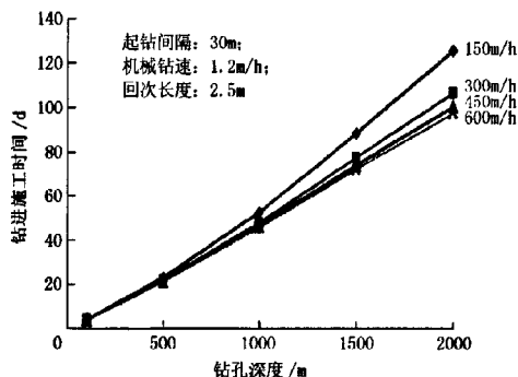
图4 起下钻速度对钻进施工时间的影响
