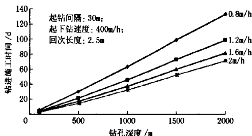
图2 机械钻速对钻进施工时间的影响
