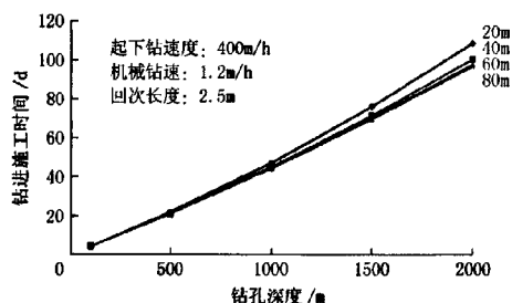
图3 起钻间隔对钻进施工时间的影响
