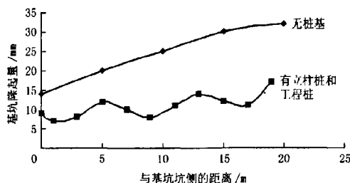
图6 有无桩基基坑坑底隆起的变形图
