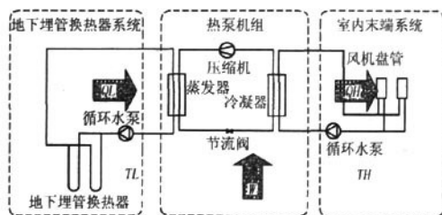
图1 供暖工况下地源热泵系统运行原理示意图
