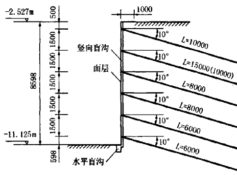
图2 基坑北面围护剖面图
