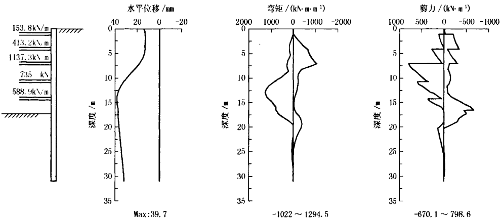
图 2 基坑变形及受力计算结果
