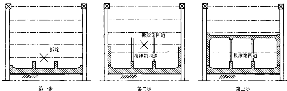
图1 施工工序示意图
