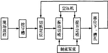
图 3 振动切喷工艺流程图
