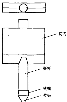
图1 振动切喷钻具图
