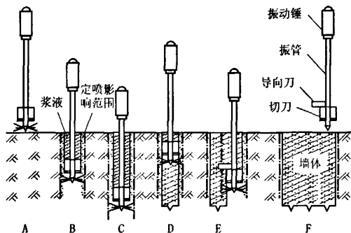
图2 振动切喷防渗墙施工原理图
