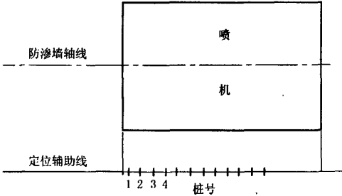
图 4 振动切喷辅助线定位放样图
