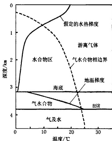
图1 天然气水合物压力(深度)和温度稳定区间图
