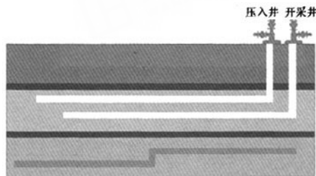
图5 打开采井并加长水平井段的长度
