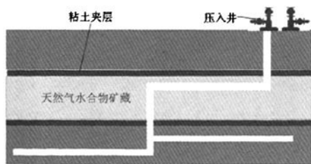
图2 向天然气水合物地层钻压入井
