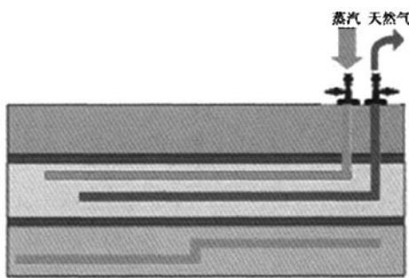
图6 向压入井注入蒸汽,增加储层渗透性,在产气储层中形成天然气
