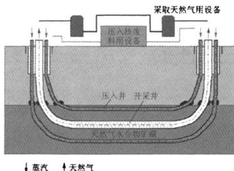
图8 利用双井筒大水平距对接智能井开采天然气水合物
