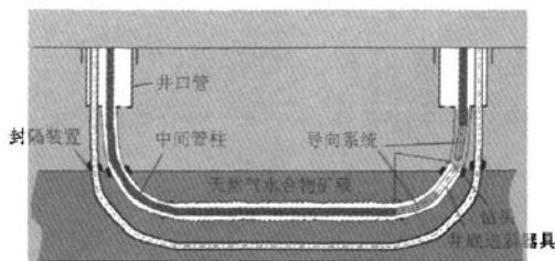
图7 利用导向系统和造斜系统钻进双井筒大水平距对接智能井
