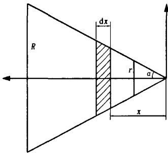
图2 挤压式钻头模型
