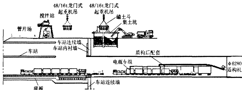
图1 地铁隧道区间土压平衡式盾构机掘进示意图
