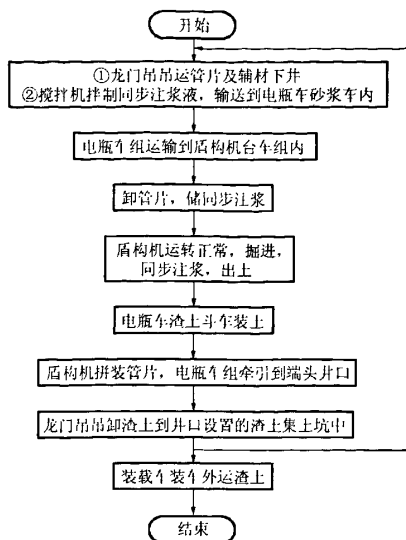
图2 单环掘进施工工序流程图
