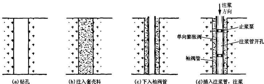
图2 袖阀管注浆及结构示意图
