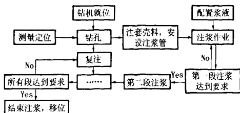
图1 袖阀管注浆工艺流程图
