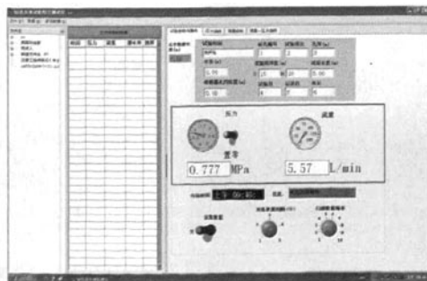
图3 钻孔压水试验测试仪电脑操作界面
