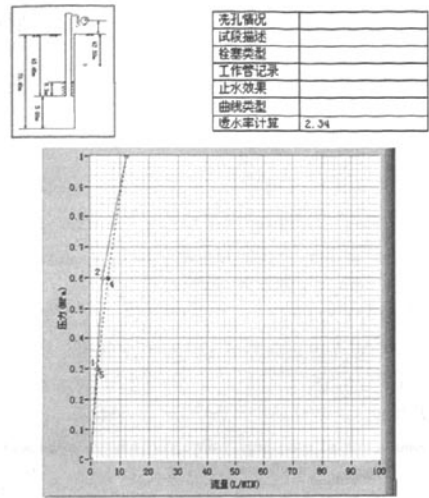
图6 仪器自动生成的 P-Q 曲线
