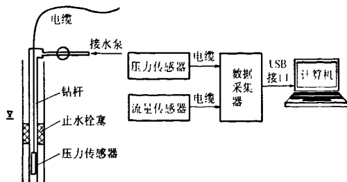
图2 工作原理示意图
