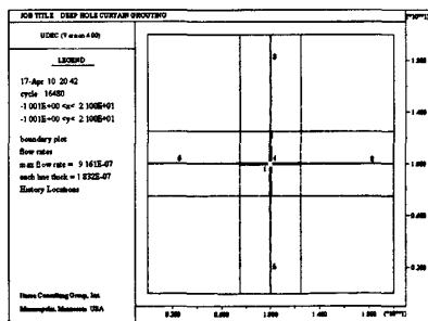
图10 P = 6.5 MPa时浆液流动扩散图
