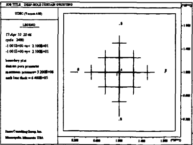
图2 P = 3.2 \text{ MPa} 时裂隙灌浆压力分布
