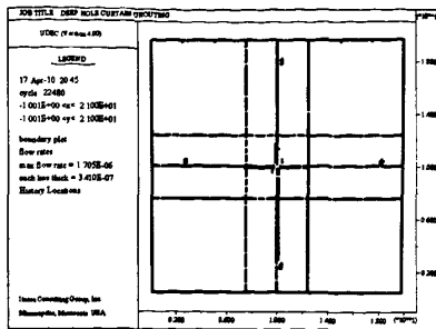
图12 P = 8.0 MPa时浆液流动扩散图
