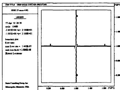
图9 P = 5.0 MPa时浆液流动扩散图
