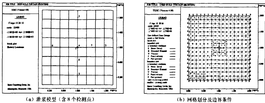
图1 UDEC 帷幕灌浆数值模拟建模界面
