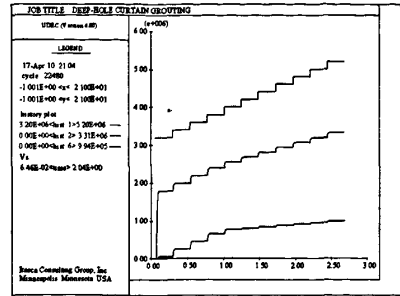
图7 hist 1、hist 2 及 hist 3 处灌浆压力曲线
