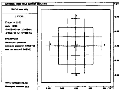
图5 P = 7.0 MPa 时裂隙灌浆压力分布
