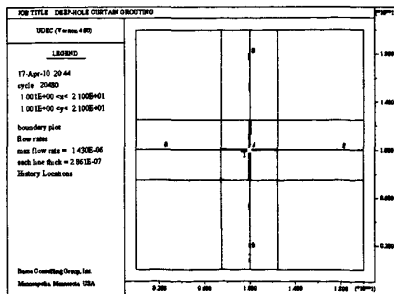
图11 P = 7.5 MPa时浆液流动扩散图
