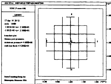
图4 P = 6.5 MPa 时裂隙灌浆压力分布
