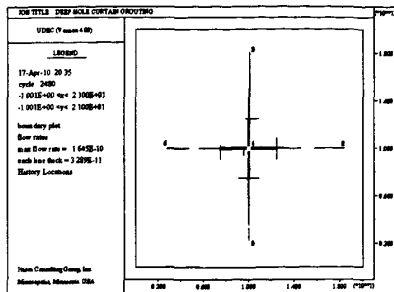
图8 P = 3.2 MPa时浆液流动扩散图
