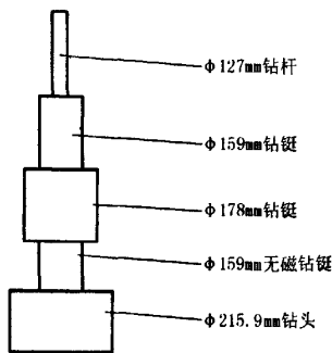
图2 钻具组合示意图
