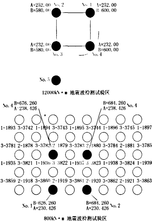
图2 12000和8000 kN·m强夯振动测试平面布置图
