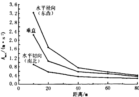
图4 12000 kN·m 测试成果曲线图
