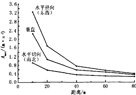
图3 8000 kN·m 测试成果曲线图
