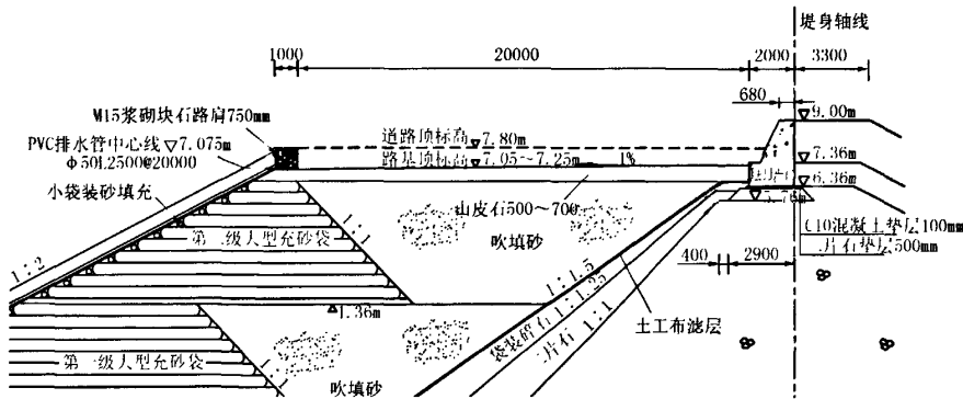
图1 海堤与地基处理区域的相对位置图
