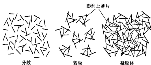
图2 膨润土泥浆触变性示意图
