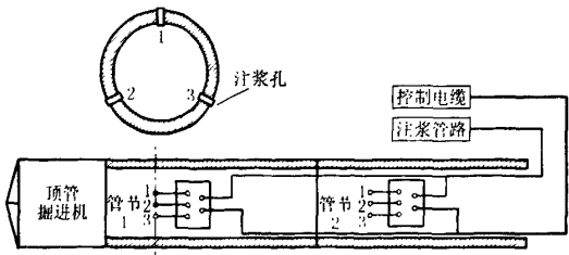
图 5 注浆系统示意图
