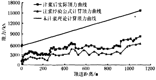
图 6 顶力与顶进距离关系图
