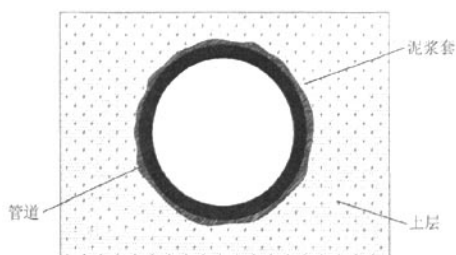
图4 泥浆与土体形成泥浆套
