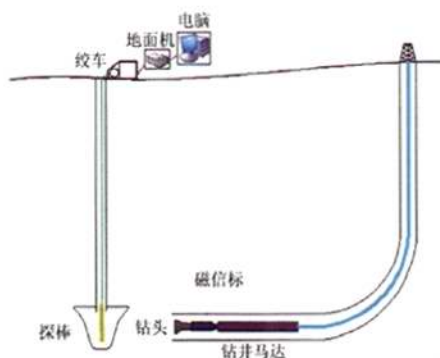
图 1 SmartMag 测井示意图
