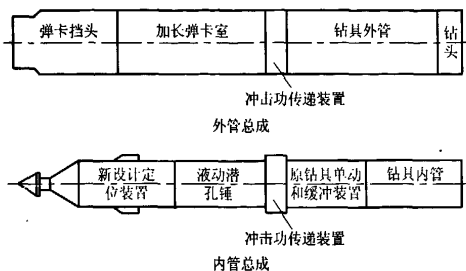
图4 改进后外管总成、内管总成结构示意图
