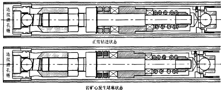
图6 钻具改进后正常工作状态和岩矿心发生堵塞状态
