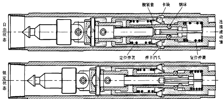
图5 定位器示意图
