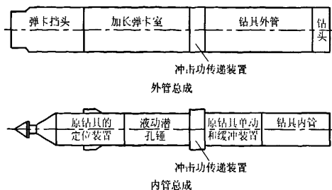
图1 外管总成、内管总成结构示意图
