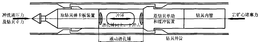
图2 内管总成“漂浮”示意图
