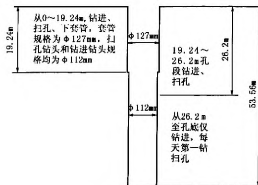
图3 钻孔孔身结构图
