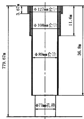
图 1 ZK4005 号钻孔结构示意图
