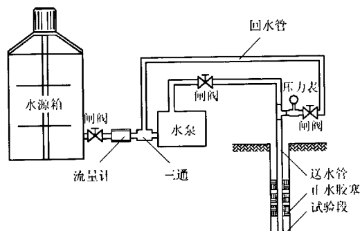
图 2 压水试验管路安装示意图
