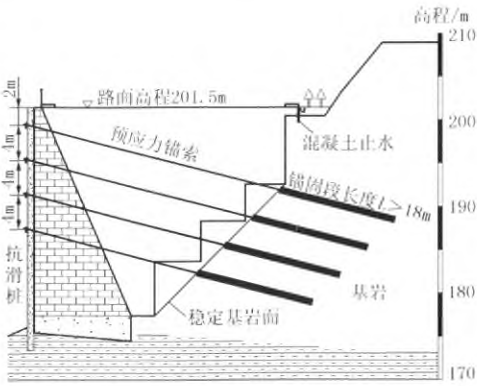
图2 预应力加固结构断面图
