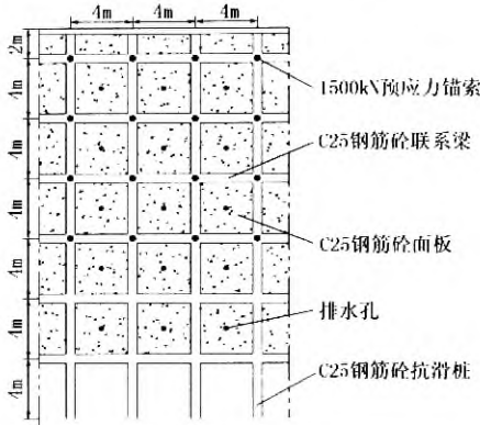
图3 预应力加固结构立面图
