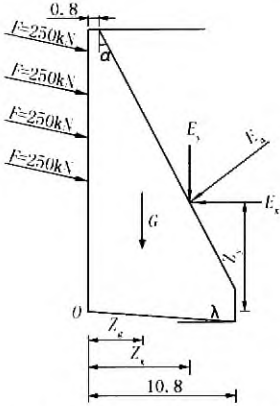
图4 作用于挡土墙的力系图(每延米)
