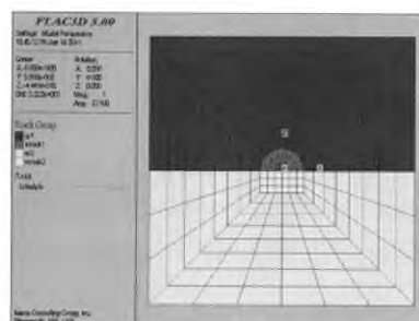
图2 试验洞 FLAC 3D 计算模型
