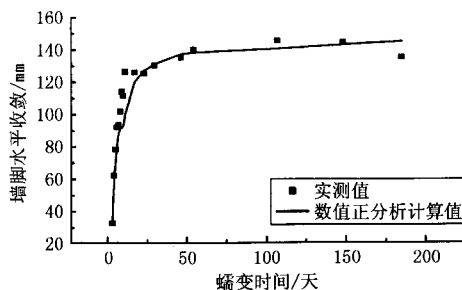
图 16 墙腰水平收敛实测值与数值正分析值对比图
