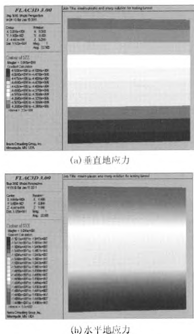
图3 初始地应力云图
