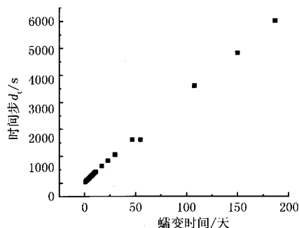
(a) 计算拱脚位置水平收敛时
