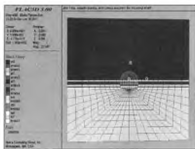
图 12 隧道 FLAC 3D 计算模型
