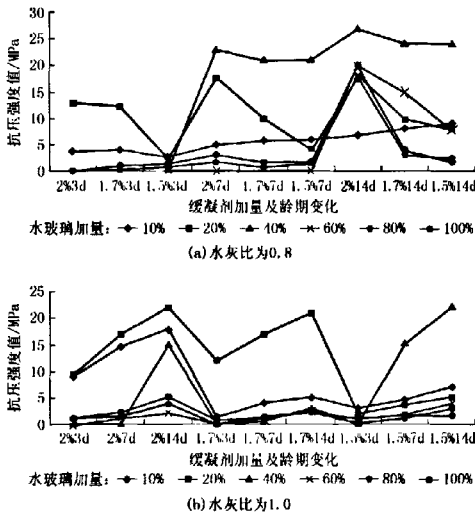
图4 磷酸氢二钠加量对水泥-水玻璃结石体抗压强度的影响
