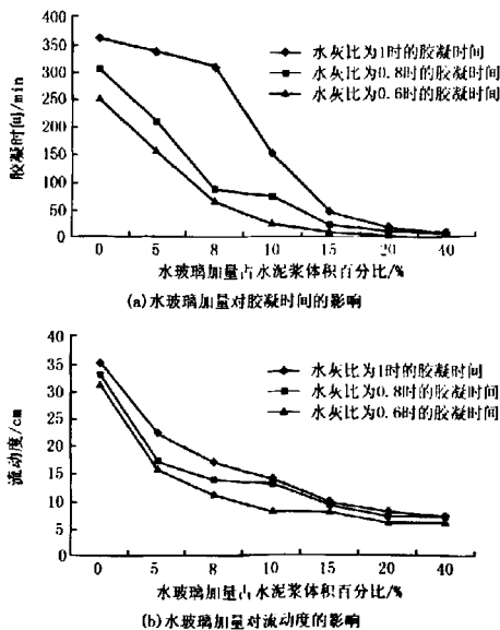
图1 水泥-水玻璃浆液凝固特性试验结果
