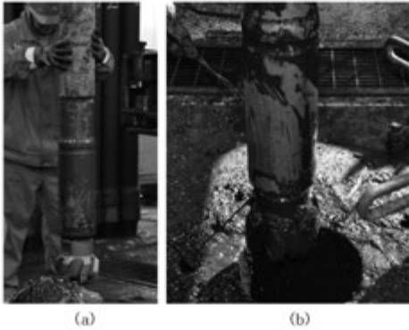
图 4 扭力冲击器入井和出井照片
