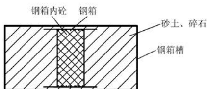
图4 钢箱两侧回填及内部浇砼示意图
