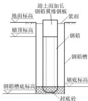
图3 钢箱封底状态示意图
