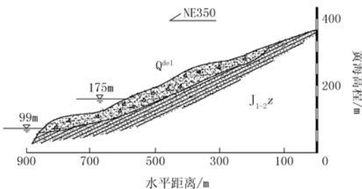
图 2 黄莲树滑体监测剖面图
