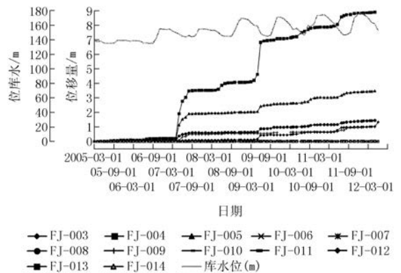
图 3 黄莲树滑坡 GPS 监测点矢量位移时间曲线图
