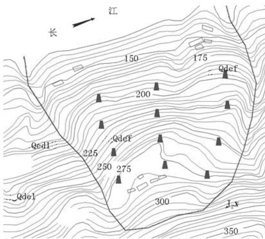
图 1 黄莲树滑体监测预警平面布置图
