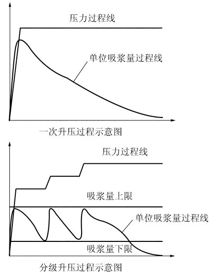
图 1 升压过程示意图
