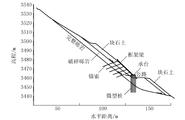
图 1 滑坡治理工程措施示意图
