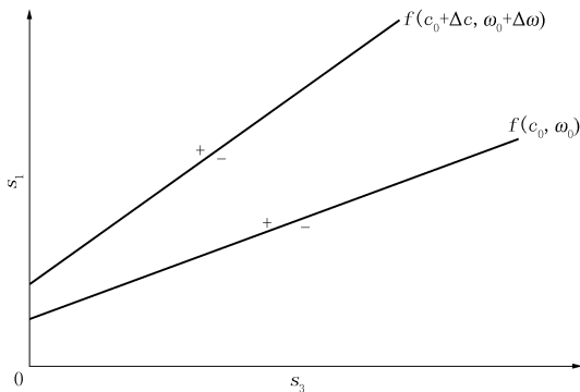
图3 Mohr-Coulomb 屈服准则
