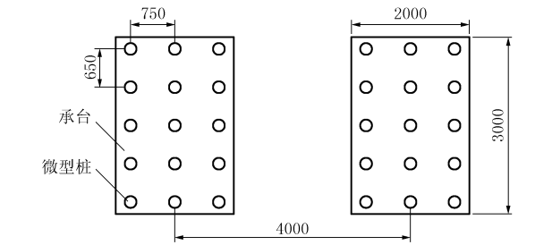
图 2 微型组合抗滑桩布置示意图
