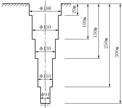
图 2 钻孔结构设计图
