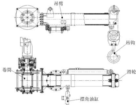
图3 液压吊车组件示意图
