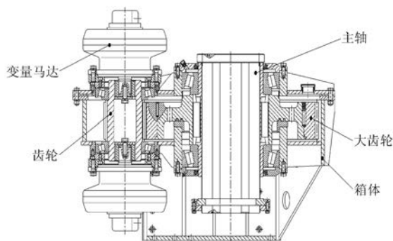
图2 全液压力头结构示意图
