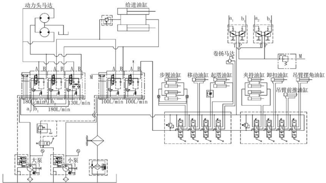
图4 液压系统示意图
