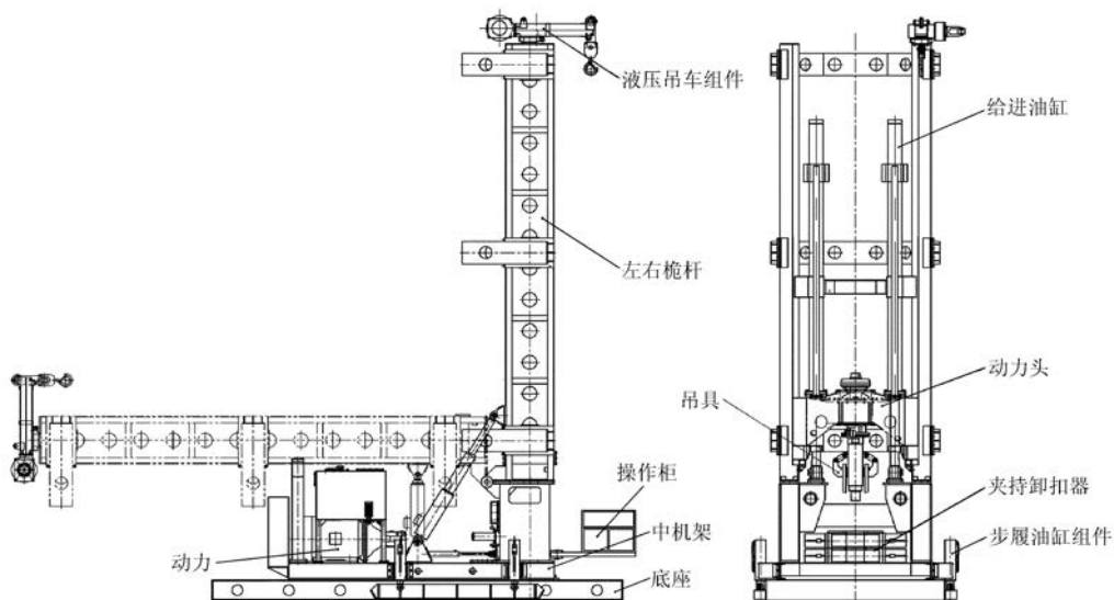
图1 GYD-20 型钻机装配图
