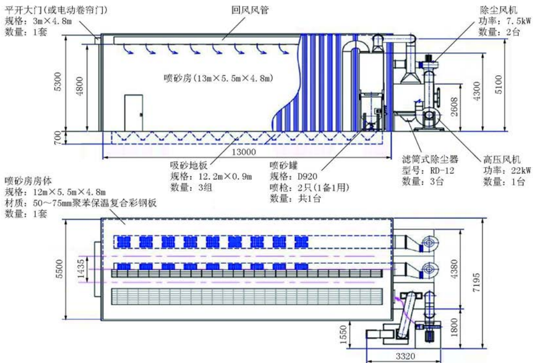
图1 PSF 13 \text{ m} \times 5.5 \text{ m} \times 4.8 \text{ m} 喷砂房设备安装图
