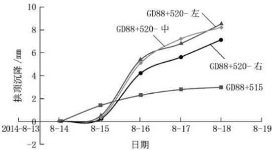
图 7 拱顶累积沉降量
