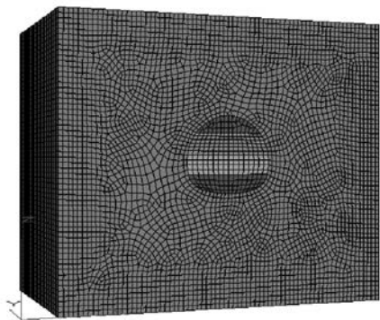
图 5 三台阶开挖计算模型
