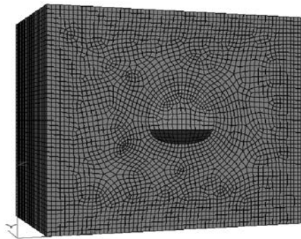
图 4 全断面开挖计算模型
