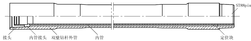
图 1 双壁钻具基本结构
