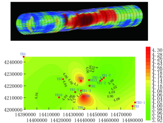
图 1 麦盖提玉北 6 井套管挤毁成像测井图及异常地应力分布规律图
