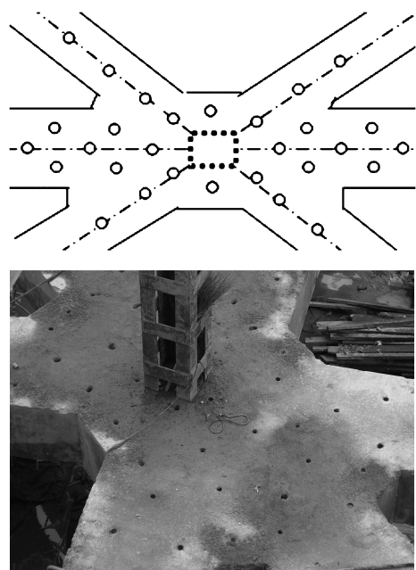
图 5 节点布孔示意
