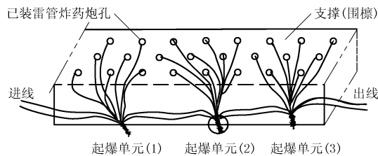
图 6 起爆网络示意图
