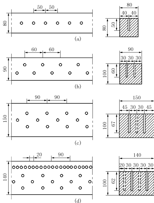
图4 典型支撑与围檩布孔示意图
