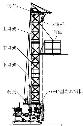
图1 塔机一体钻机结构示意图
