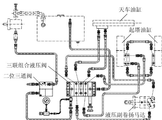
图4 液压管路图
