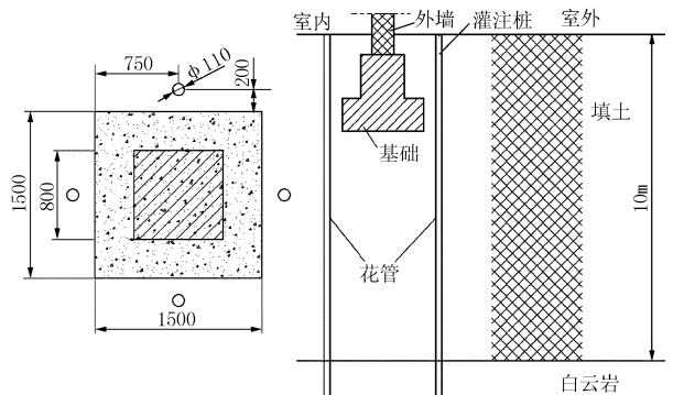
图4 钻孔布置及剖面图
