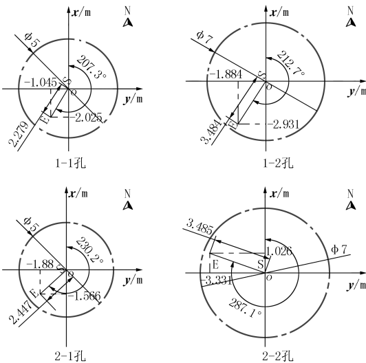
图 14 充填孔终孔坐标位置示意图
