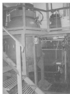
(a) 内部容积为 2\text{m}^3 的爆炸腔室
