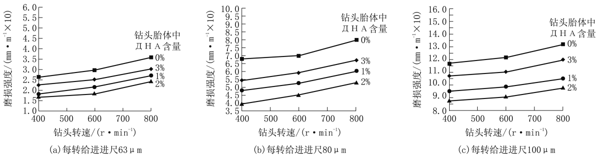
图3 不同转速、每转不同进尺时, 磨损强度与钻头胎体中 ДHA 含量的关系曲线
