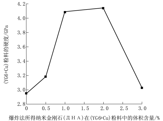
图2 金刚石钻头胎体材料(YG+Cu)硬度与胎体中 ДHA 含量的关系
