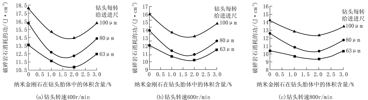
图4 不同转速、每转不同进尺时, 破碎单位体积科罗斯德舍夫花岗岩消耗的功与钻头胎体中 ДHA 含量的关系曲线
