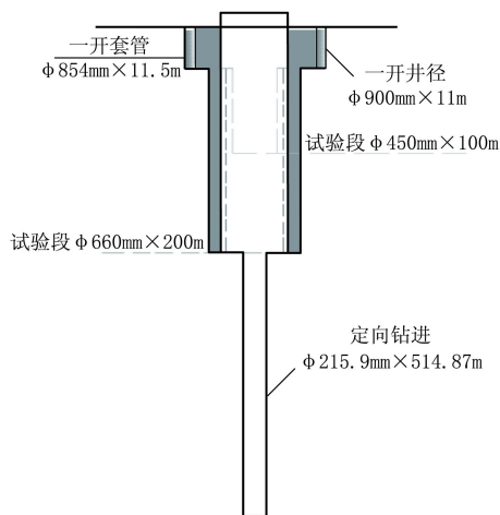
图 1 实际井身结构示意图
