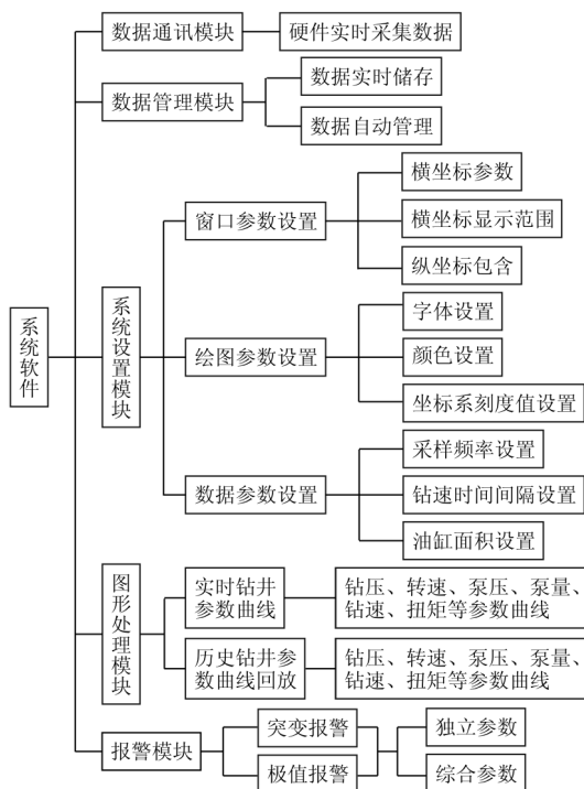
图 3 系统软件功能模块组成
