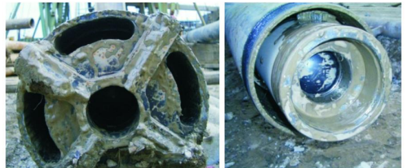
图13 保压取心钻具试验现场及球阀关闭情况
