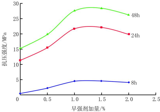
图 2 M59S 加量与水泥石强度的变化关系
