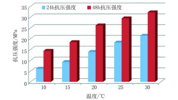
图 4 不同温度下水泥石抗压强度变化情况
