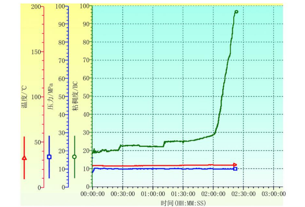
图 3 低温早强水泥浆稠化曲线
