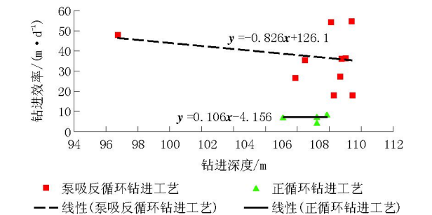
图 6 正循环钻进和泵吸反循环钻进效率趋势图
