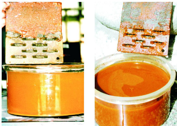
图2 普通钢管—镀锌桥式管电偶腐蚀挂片试验
