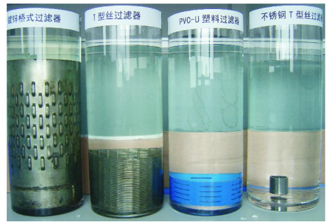
图3 不同材质腐蚀结垢试验
