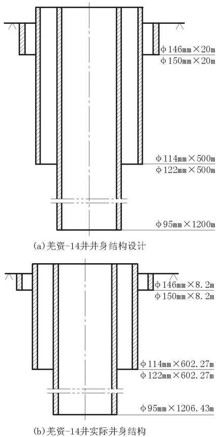
图 1 羌资-14 井井身结构图
