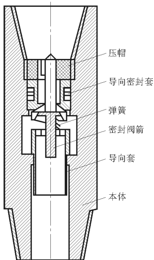
图2 箭形回压阀
