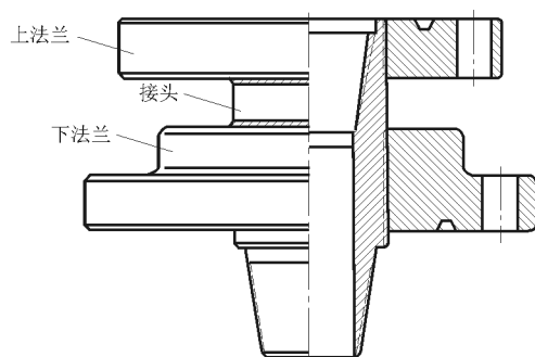
图5 压酸钻杆挂
