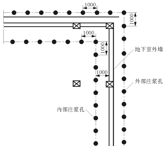
图 3 注浆方案图
