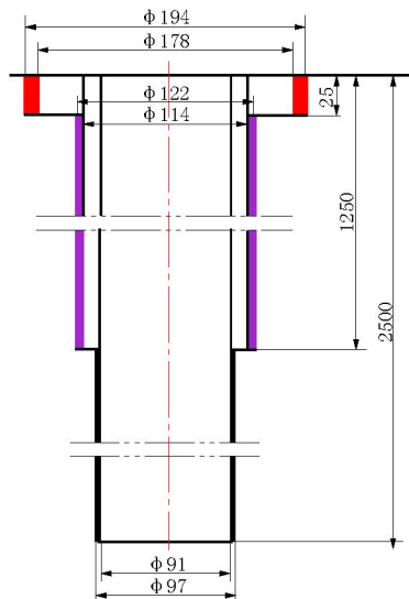
图 1 “羊 D1”钻井井身结构示意图
