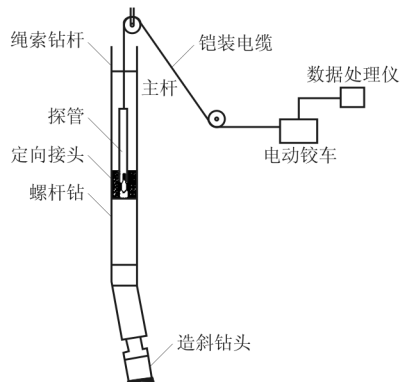
图 1 定向系统
