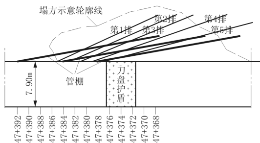
图4 管棚及灌浆孔布置示意图
