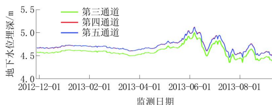
图12 D5多层监测数据曲线
