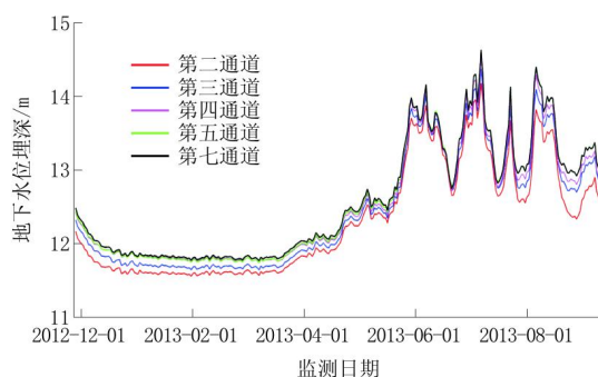
图11 D4多层监测数据曲线
